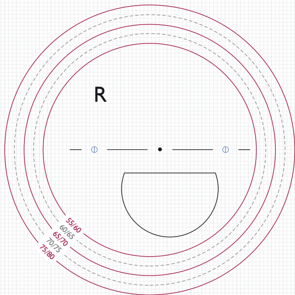
BI-FOCAL D25 (ind. 1.50)
